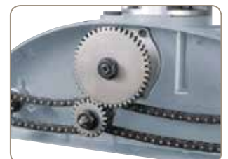
Einfacher Geschwindigkeitswechsel durch Umstecken der Zahnräder
